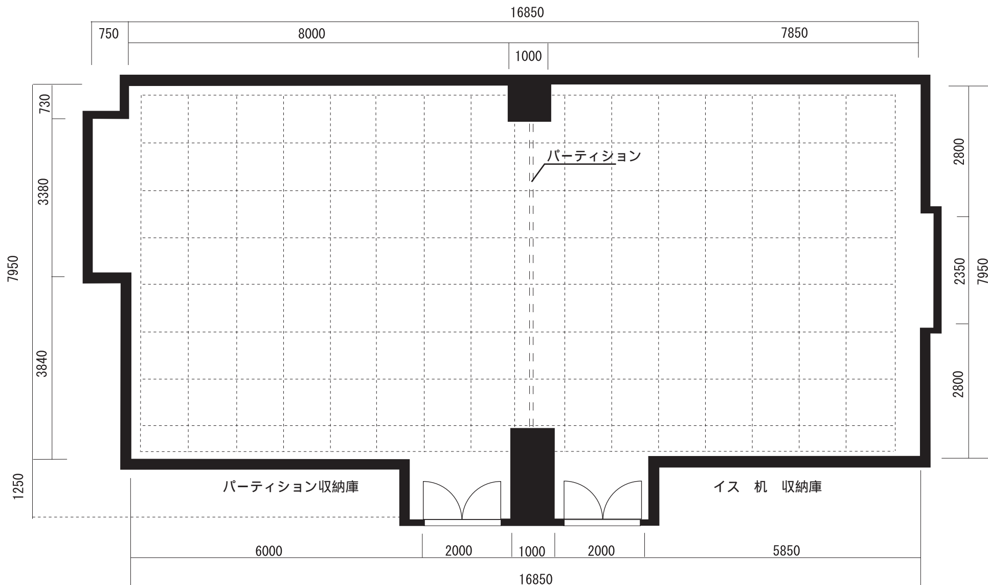
大阪府立中央図書館 大会議室 平面図 138m 2
